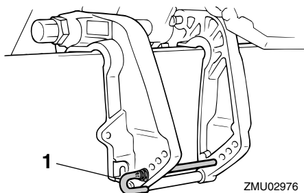
1. Trim rod
